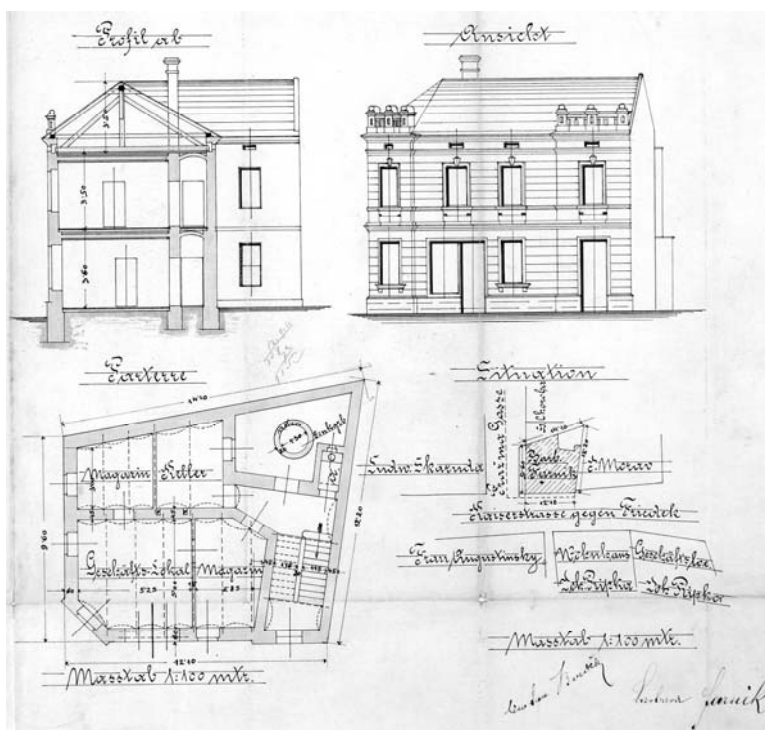
Plány domu Barbary Farnikové č. 42 na nároží ulic Tří Prutků a Pražmovy, autor A. Bezděk, rok 1903
