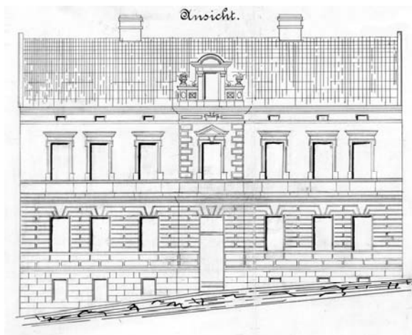
Dům p. Ullmanna č. 588 na Růžovém pahorku, autor: A. Bezděk, rok 1901
