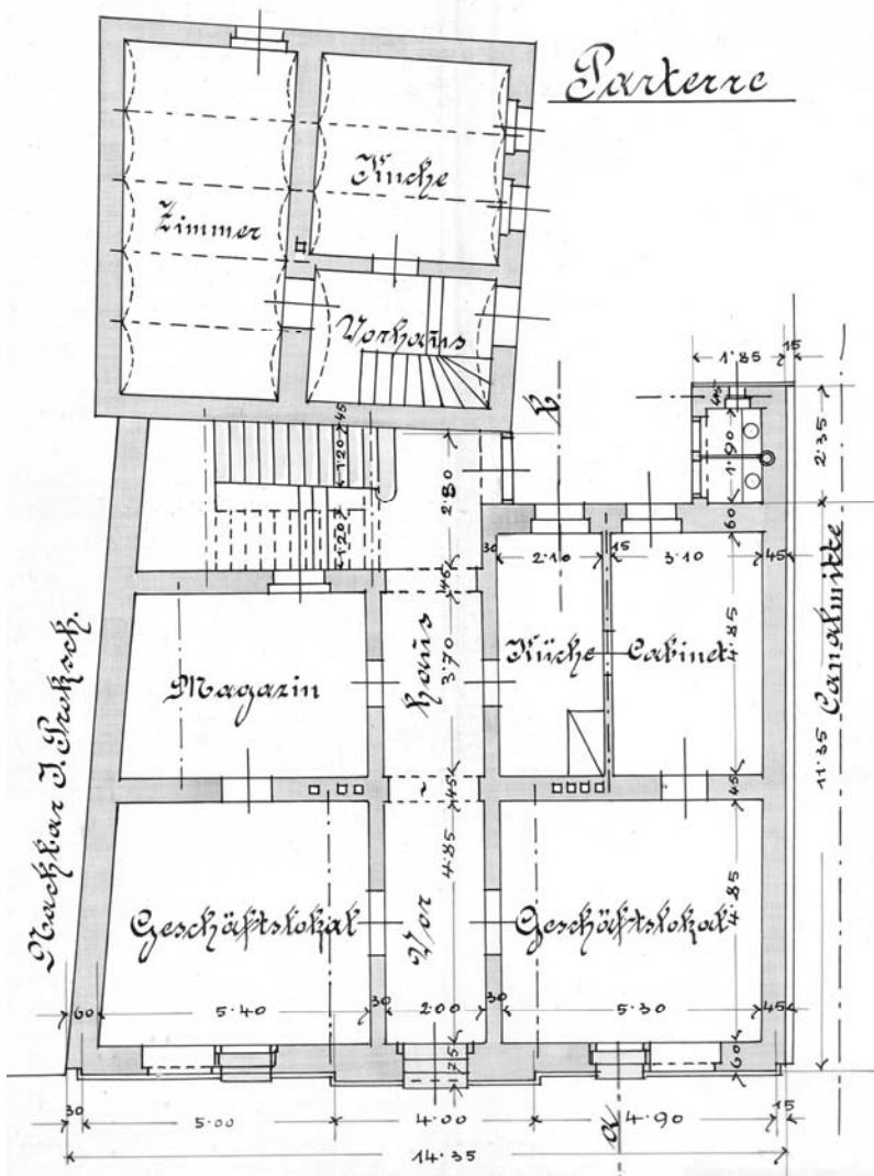
Půdorys parteru (přízemí) domu Jana Prašivky č. 38, autor: C. Fridrich, 1898
