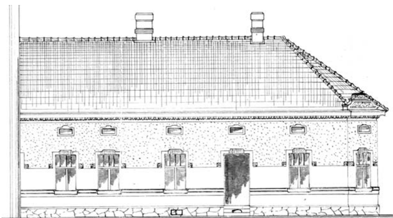
Návrh domu na parcele č. 109, autor: F. Heindrich, rok 1910
