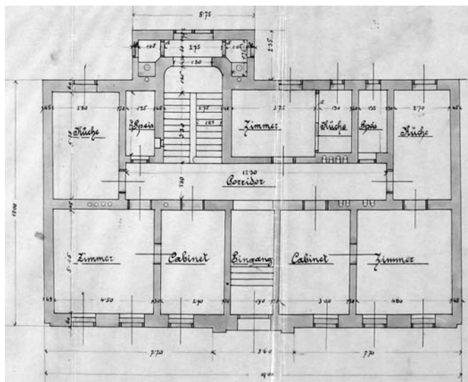
Půdorys parteru domu F. Foldiny, autor: R. Auleg, rok 1892
