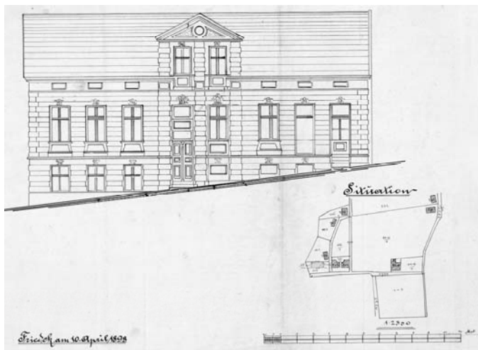
Dům p. Pomjanovského na Růžovém pahorku, autor: Hans Pohl, rok 1898
