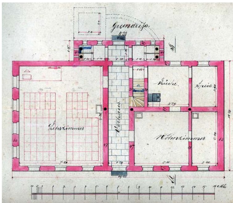
Plán školní budovy v Trojanovicích od c.k. inženýra Skalda z r. 1884
