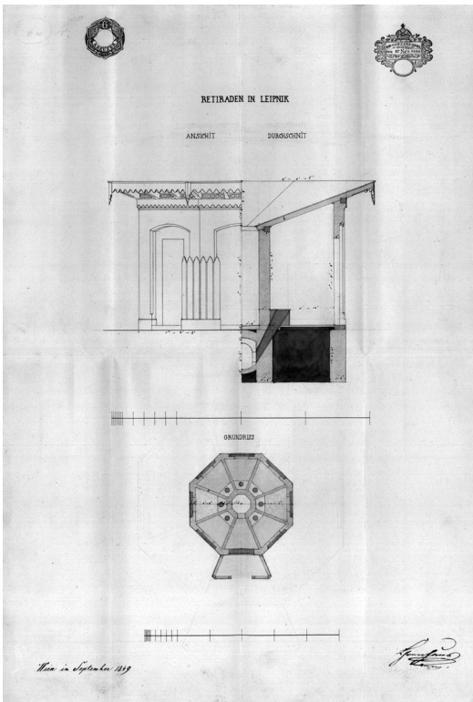
Plán záchodů z roku 1849. ZAOpO
