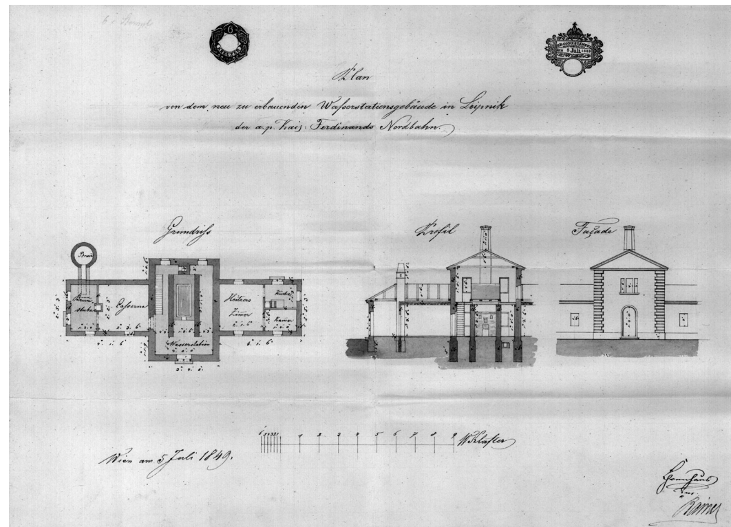
↑ Původní plán vodárny z r. 1849. ZAOpO ↓ Plán rozšíření komplexu vodárny z r. 1849. ZAOpO
