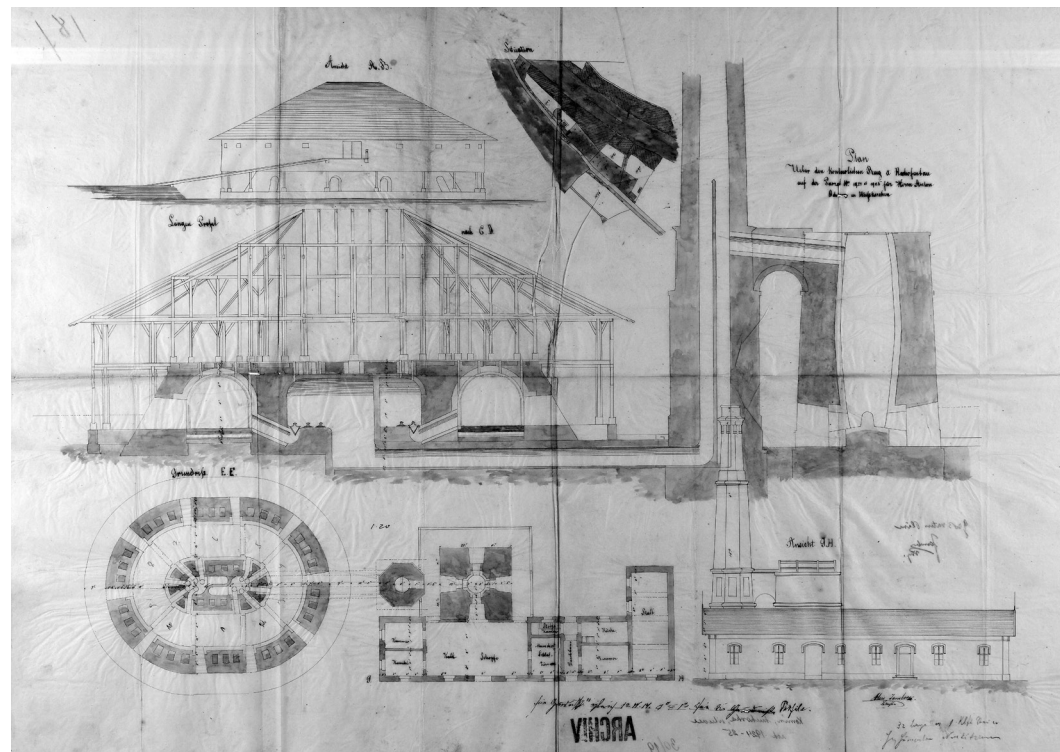
Plán na postavení kruhové pece. SOkA Přerov, fond Josef Šindler, vápenka Černotín
