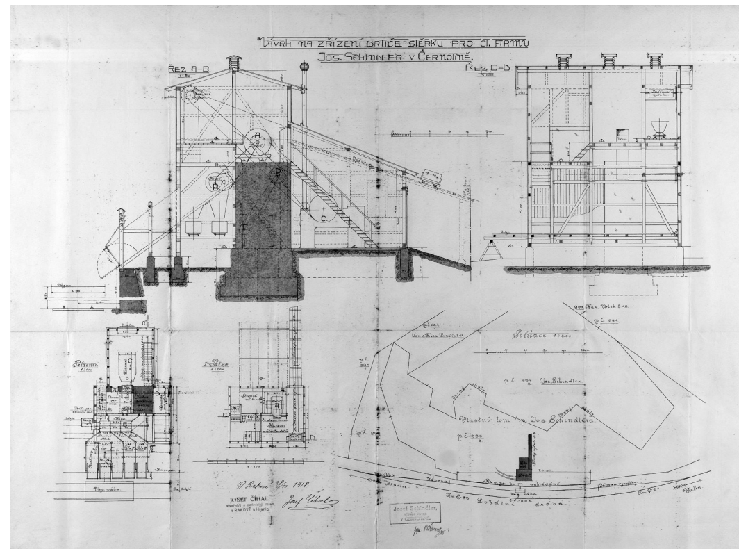
Plán na postavení drtiče šterku z roku 1918. SOkA Přerov, fond Okresní úřad Hranice
