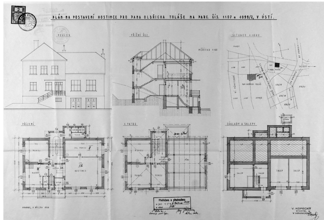
Stavební plán Oldřicha Toláše na vystavění zájezdního hostince čp. 81 v Mariánském údolí z roku 1938. SOKA Přerov, fond Okresní úřad Hranice
