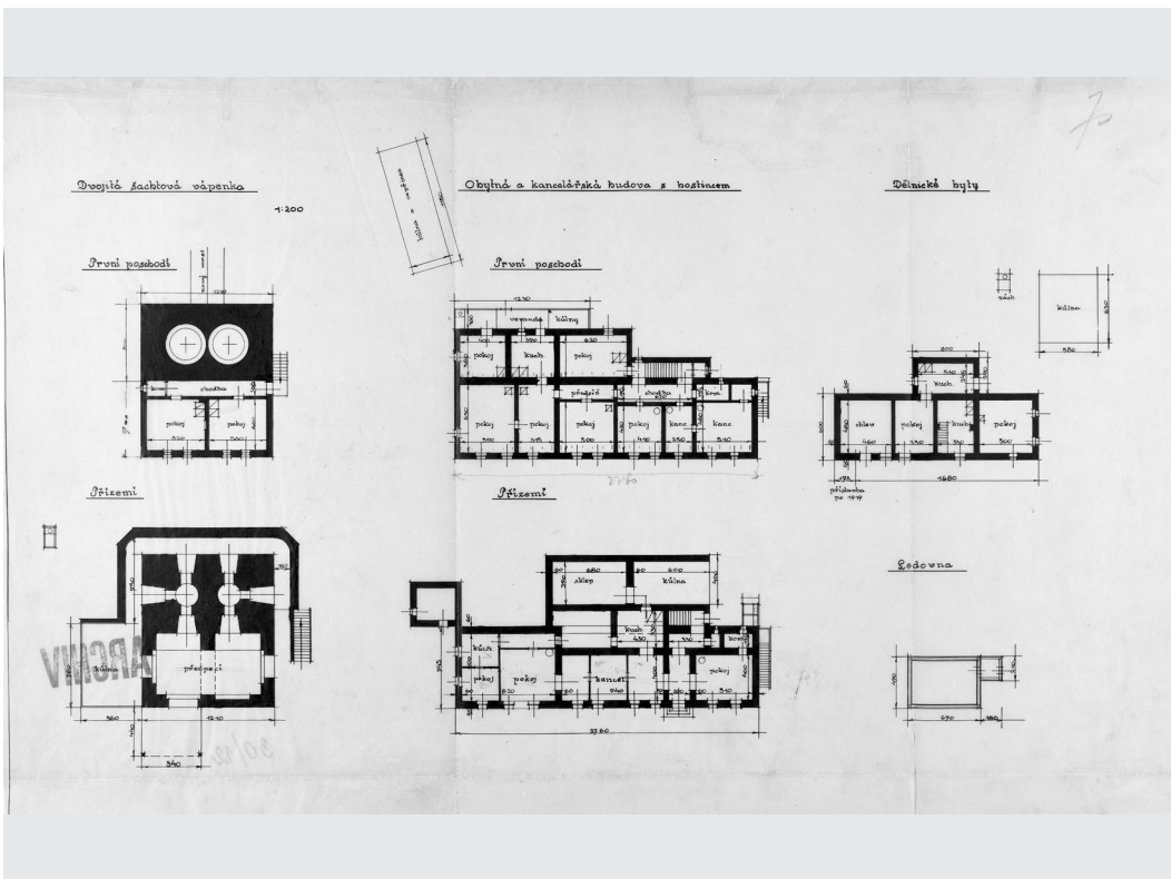
Plán dvojité šachtové vápenky, administrativní budovy, dělnických bytů a ledovny. SOkA Přerov, fond Josef Šindler, vápenka Čertotín
