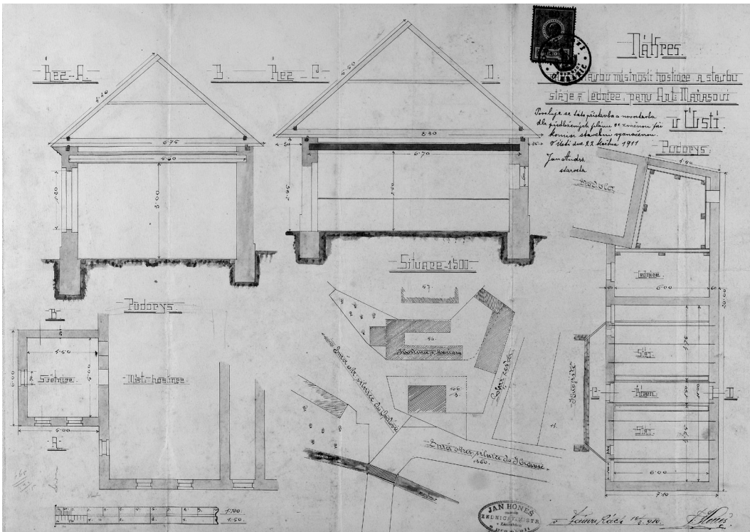
Stavební plán hostince Antonie Maňasové čp. 33 v Ústí z roku 1910. SOkA Přerov, fond Okresní úřad Hranice
