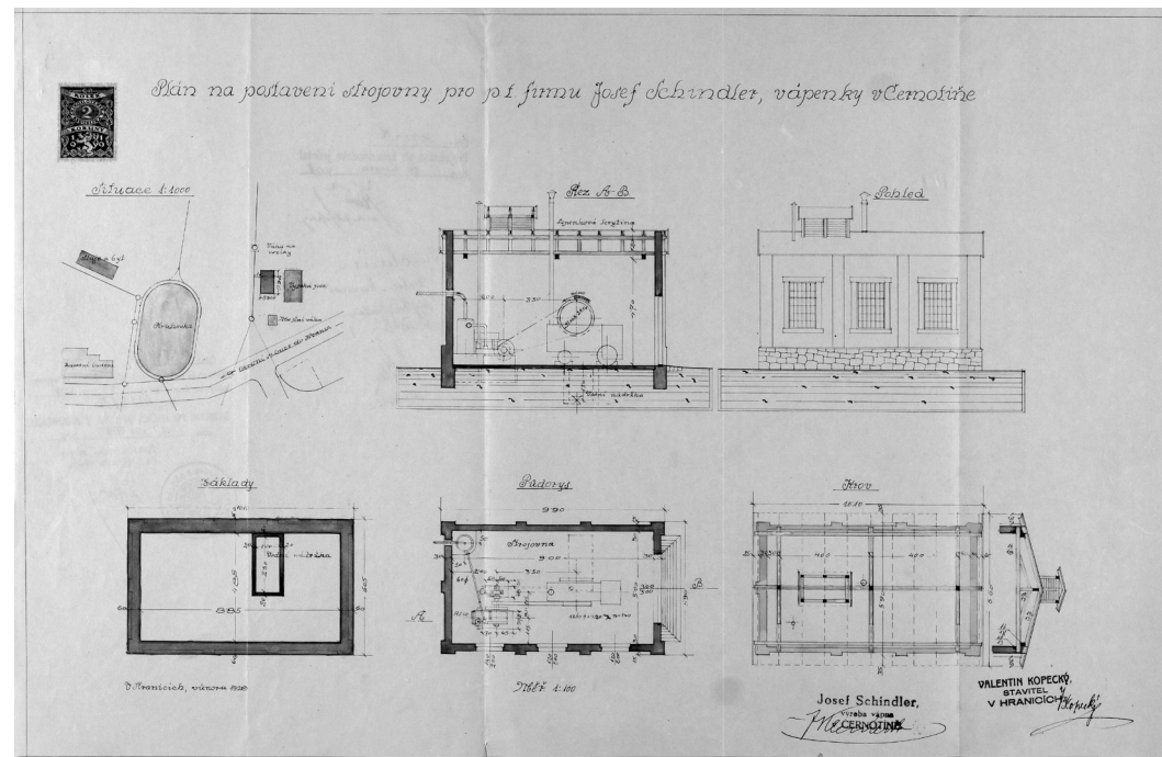
Stavební plán na postavení strojovny vedle vysoké pece z roku 1928. SOKA Přerov, fond Okresní úřad Hranice
