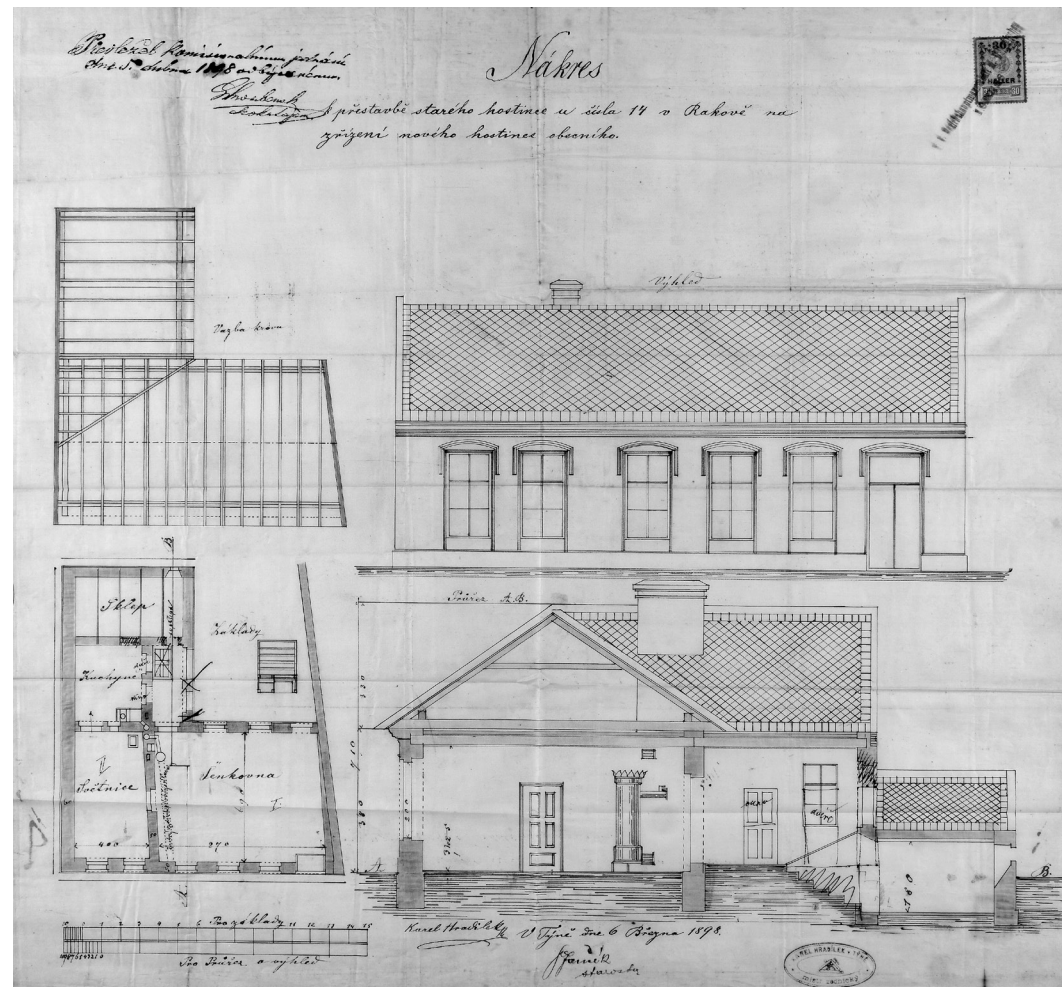
Stavební plán hostince čp. 14 v Rakově z roku 1898. SOkA Přerov, fond Okresní úřad Hranice.
