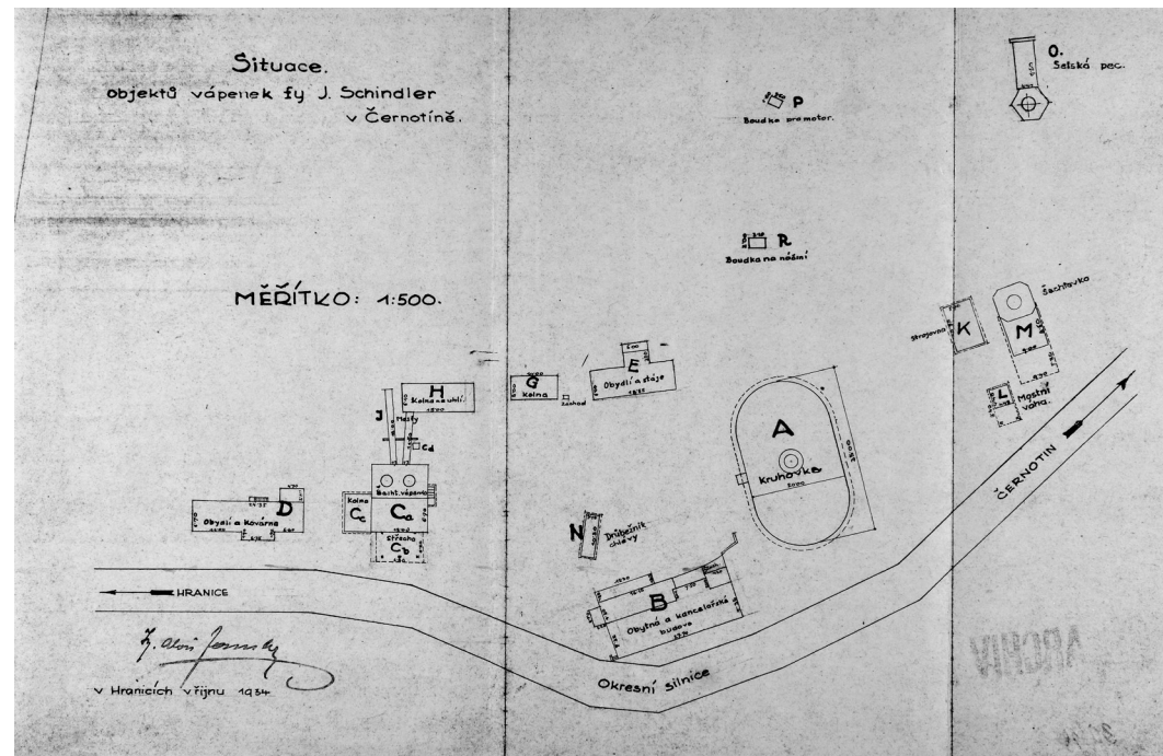
Situační náčrt objektů firmy z roku 1934. SOkA Přerov, fond Josef Šindler, vápenka Černotín
