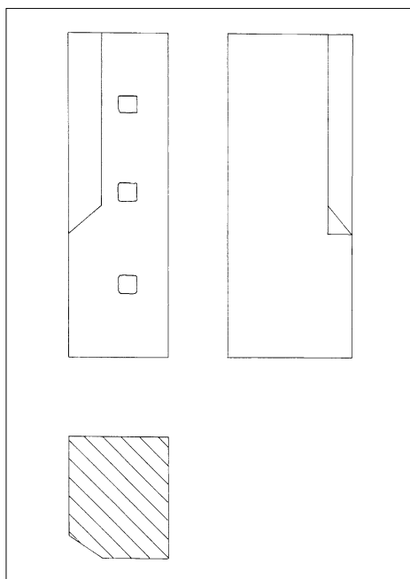
Část kamenného ostění, použitá v armování vnějšího jihozápadního nároží, nárys, bokorys, profil, 1 : 13, Z. Otruba, 1998.
