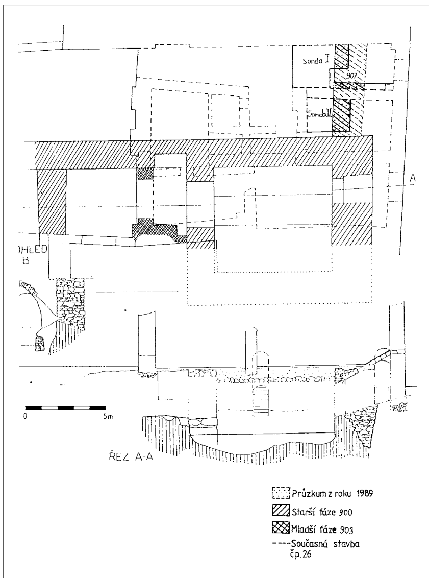
Obr. 5. Půdorys objektu č. 900 s hradbou č. 907 a vyznačením sond I a II/2000
