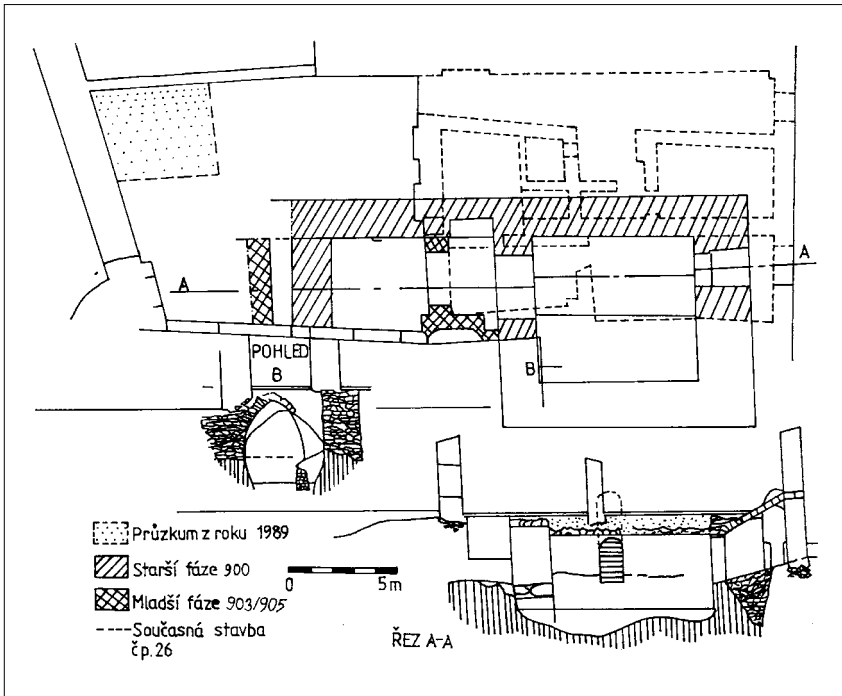
Obr. 14. Půdorys stavby č. 900 a mladší hradby č. 903–905 z pol. 15. stol.
