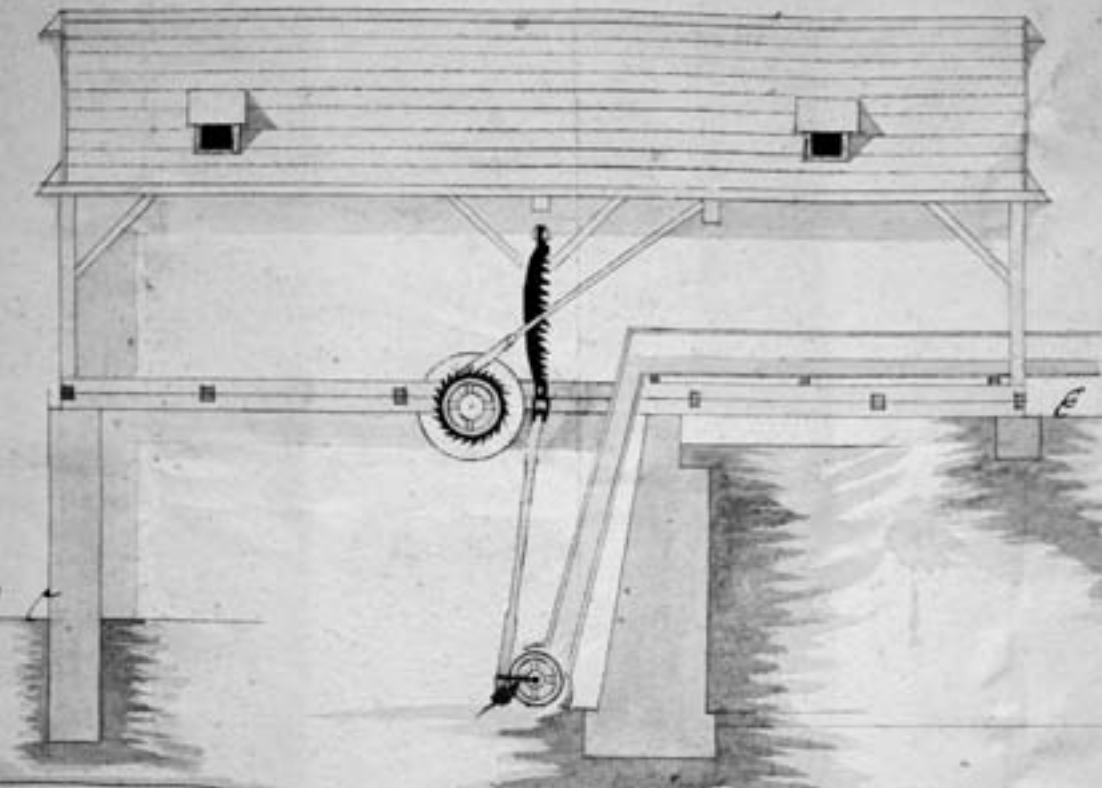
Nárys pily principu valašské jednušky mlynáře v Padesáti Lánech Josefa Klementa z roku 1821
