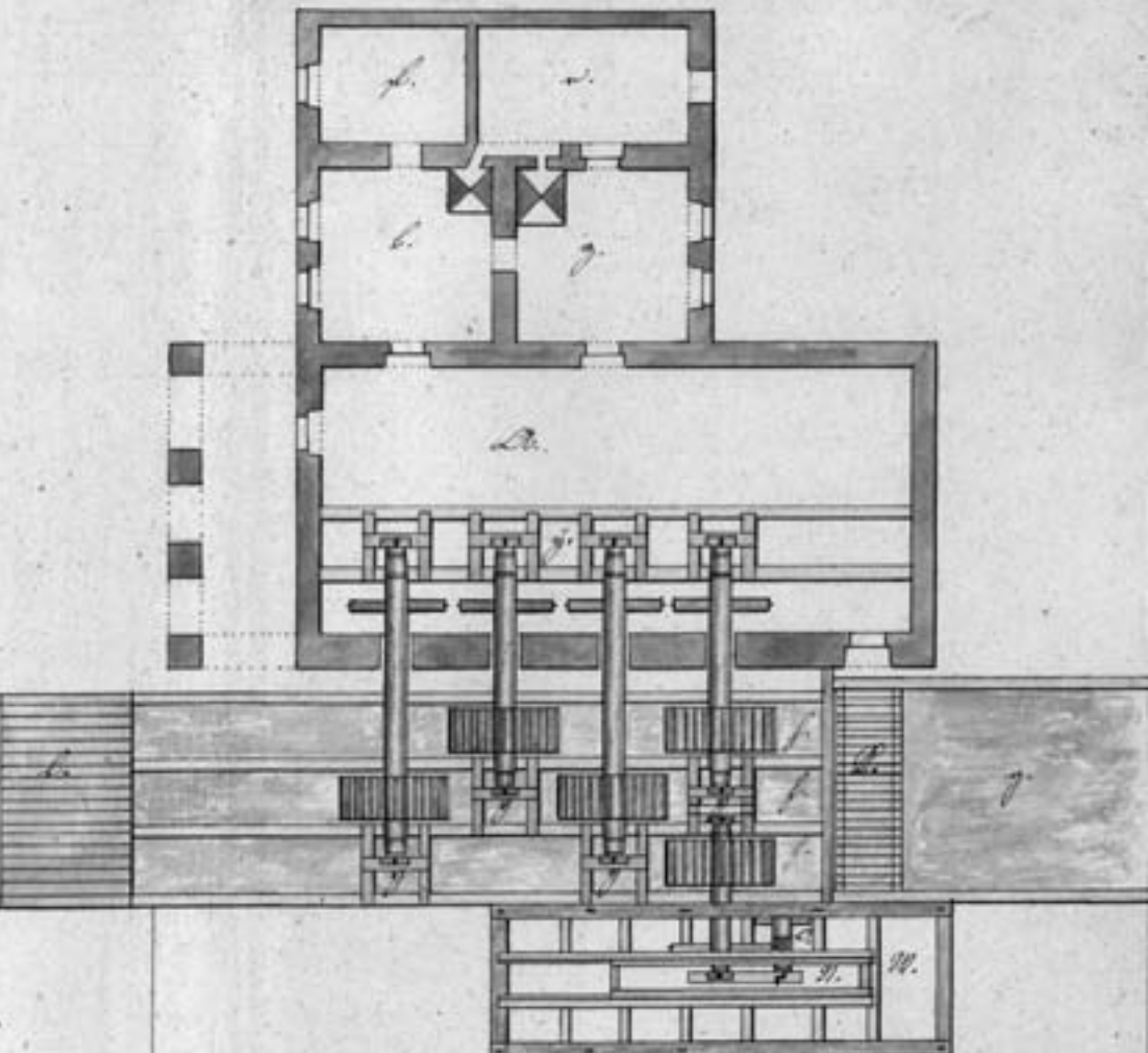
Půdorys mlýna a pily mlynáře Feylera
