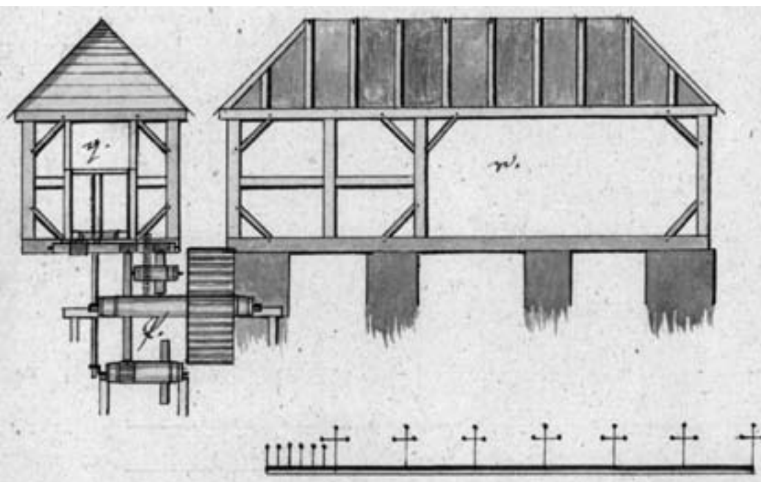
Bokorys a nárys pily mlynáře Feylera
