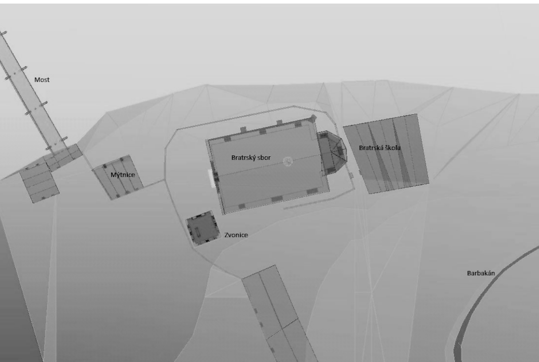
Obr. č. 6 Celková situace bratřského centra vytvořená při hmotové rekonstrukci (půdorys)
