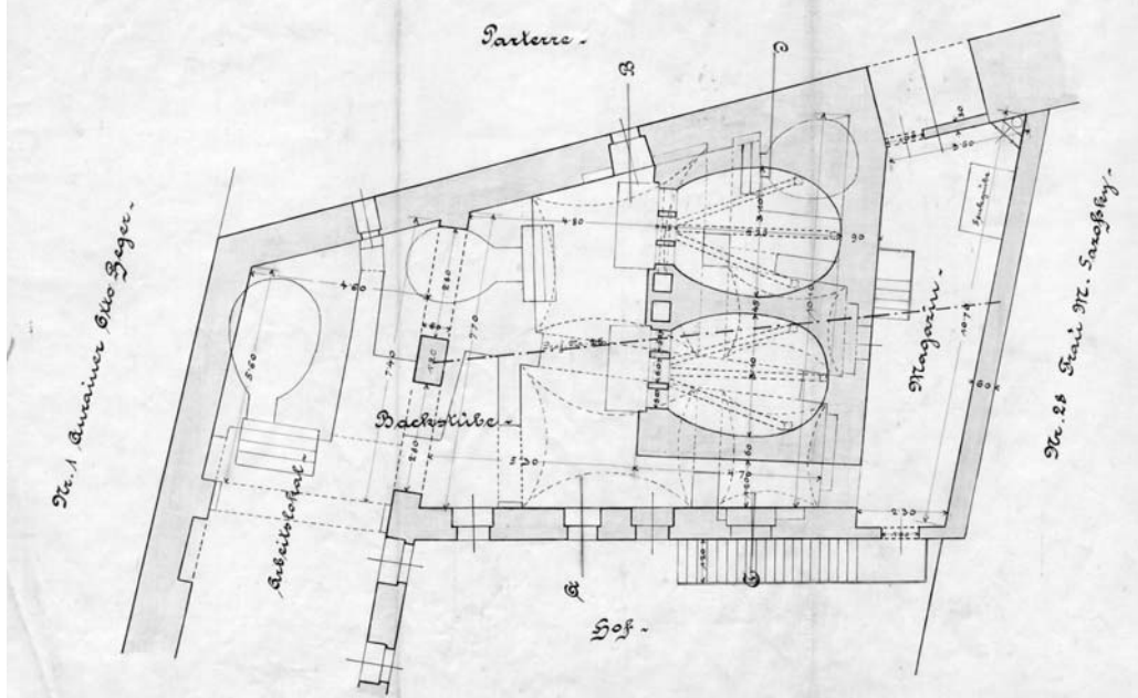
Půdorys pekárny macesů (1908)
