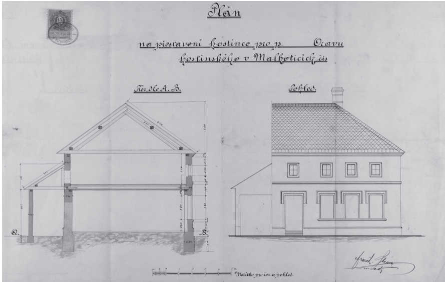
Nákres na postavení domu v Malhoticích čp. 34, hostinec u Vilímců. SOKA Přerov
