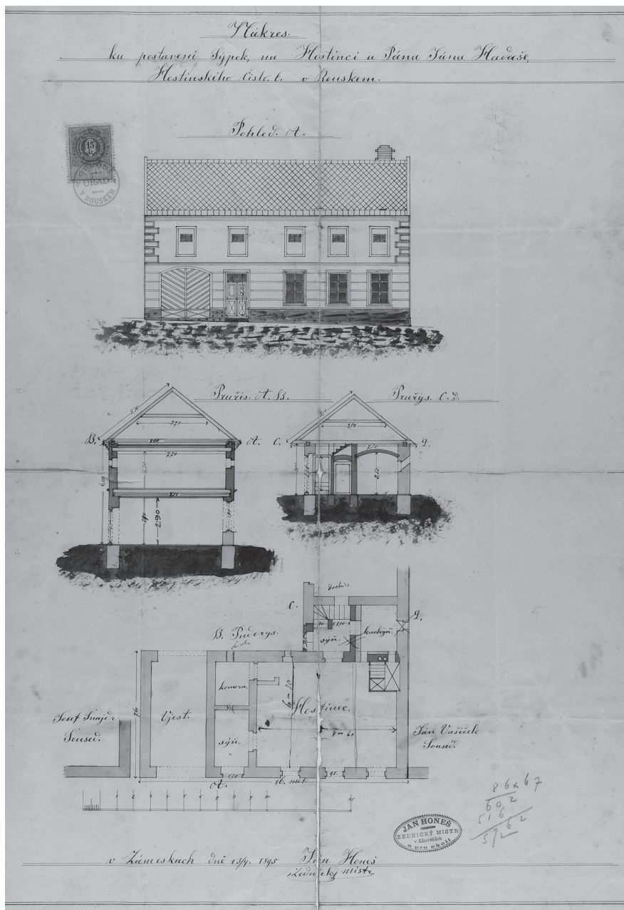
Nákres na postavení hostince Jana Hadaše, Rouské čp. 6, z roku 1895. SOkA Přerov
