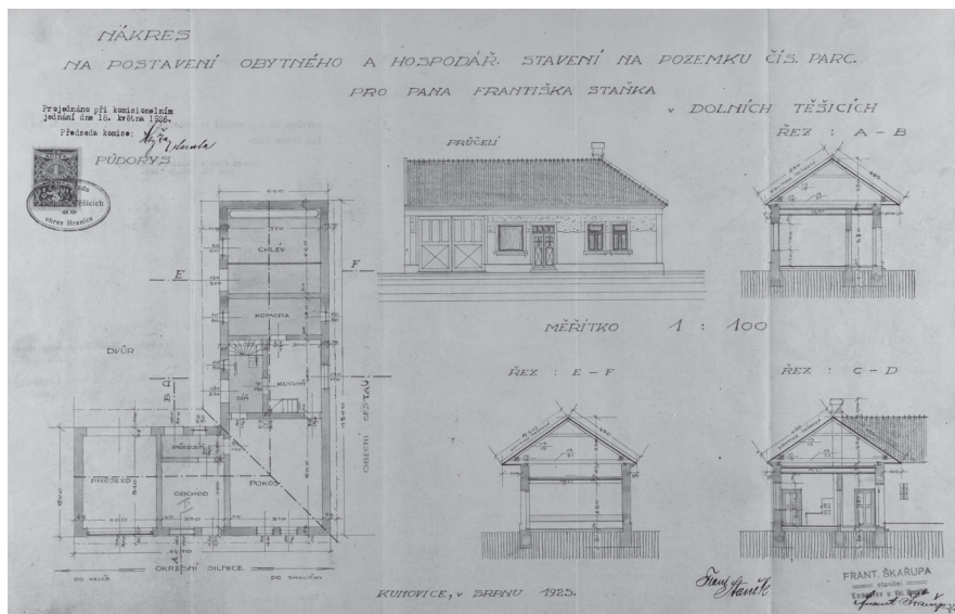
Nákres na postavení domu Františka Staňka v Dolních Těšicích z roku 1925. SOKA Přerov
