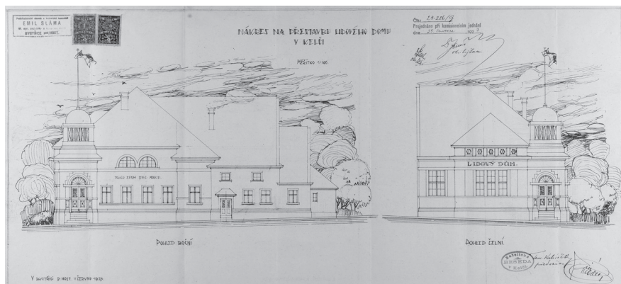
Nákres na postavení Lidového domu čp. 25 v Kelči – Posvátno z roku 1923, nyní čp. 435. SOKA Přerov
