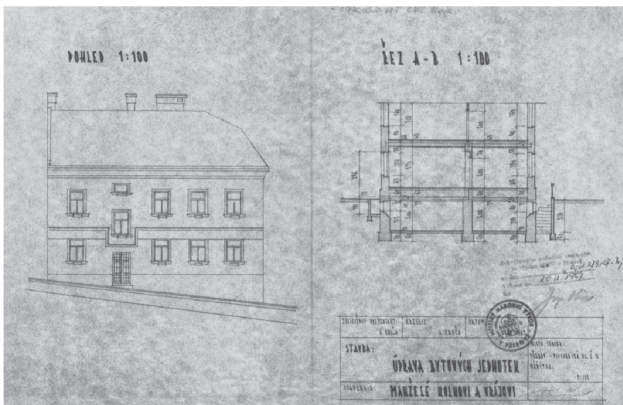
Plány projektanta Kroči z r. 1967 na úpravu fasády domu
