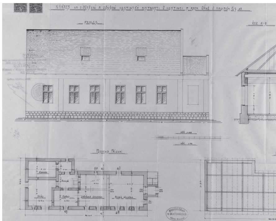
Nákrres na zvětšení a zvýšení hostinské místnosti Rajmunda Váni, hostinského v Malhoticích čp. 15. SOKA Přerov
