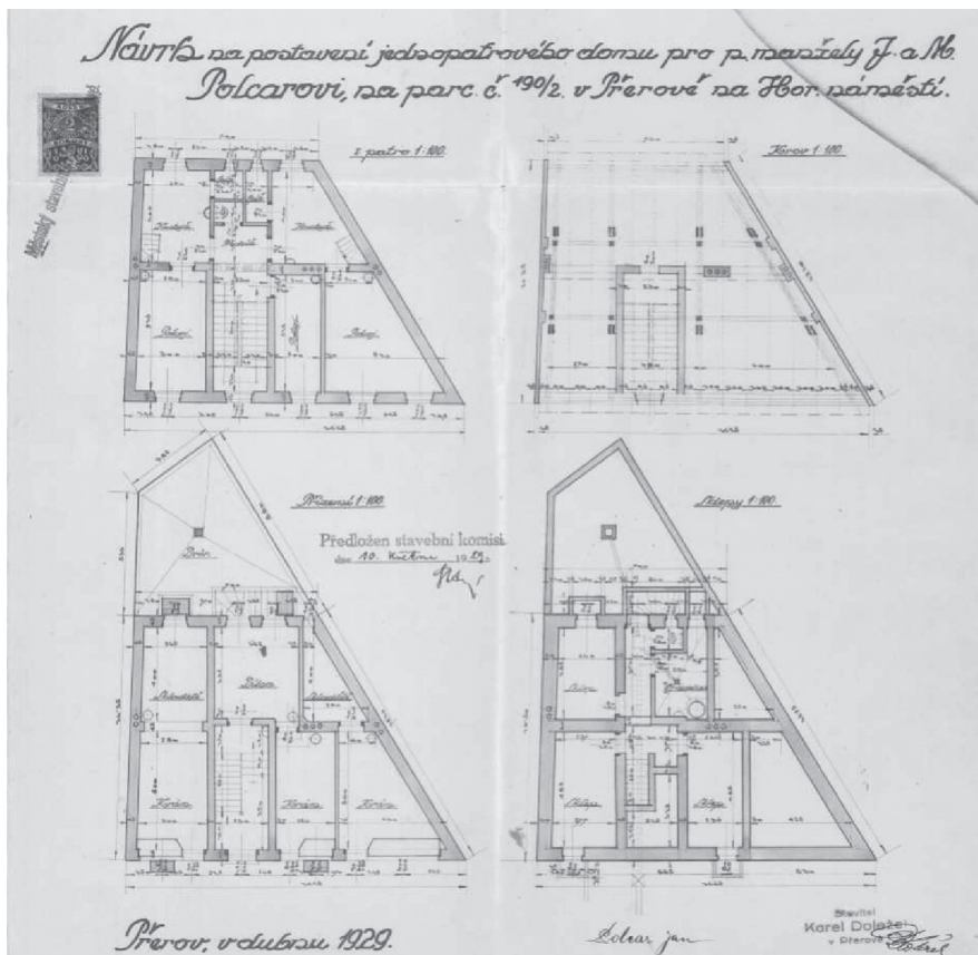
Plán k vybudování domu, autor Karel Doležel z Přerova
