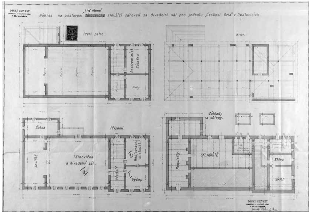
Stavební plán orlovný čp. 108 v Opatovicích. SOKA Přerov, fond Okresní úřad Hranice, inv. č. 1470, kart. č. 813
