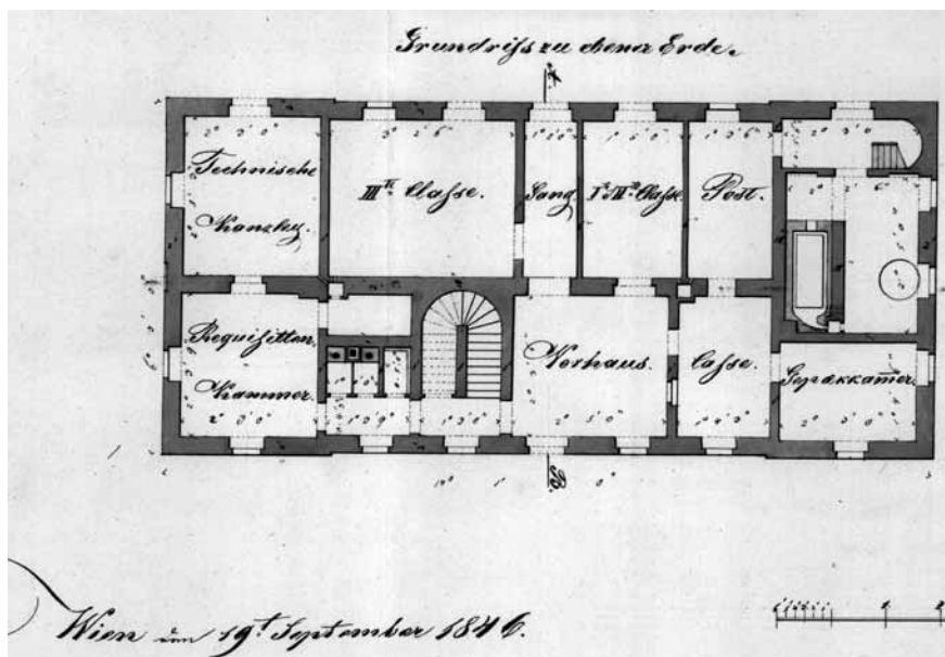
Detail plánu z roku 1846 – půdorys přízemí (ZAOpO)
