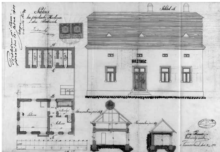
Stavební plán hostince v Babičích z roku 1903. SOkA Přerov, fond Okresní úřad Hranice, inv. č. 1445, kart. č. 793
