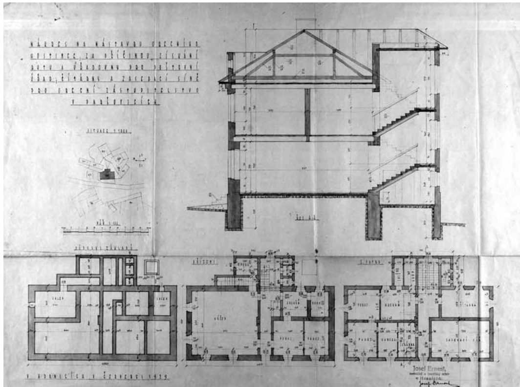
Stavební plán na přestavbu hostince čp. 32 v Paršovicích. SOkA Přerov, fond Archiv obce Paršovice, inv. č. 114
