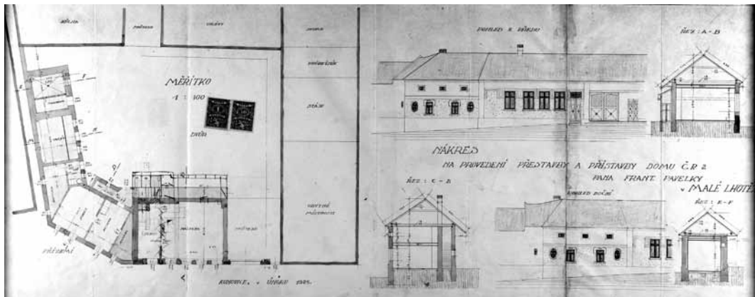
Stavební plán na přestavbu hostince čp. 2 v Lhotě u Kelče z roku 1925. SOKA Přerov, fond Okresní úřad Hranice, inv. č. 1464, kart. č. 811
