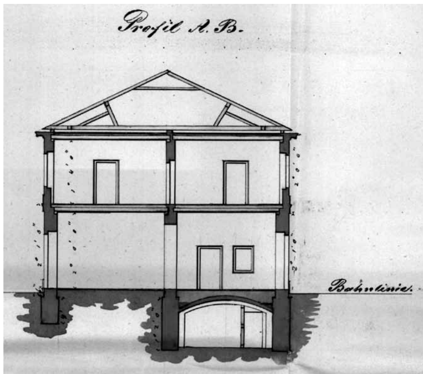
Detail plánu z roku 1846 – řez budovou (ZAOpO)
