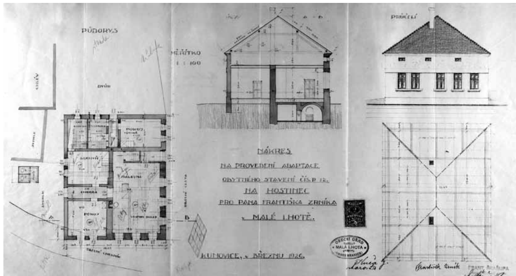
Stavební plán na přestavbu hostince čp. 12 v Lhotě u Kelče z roku 1926. SOKA Přerov, fond Okresní úřad Hranice, inv. č. 1464, kart. č. 811
