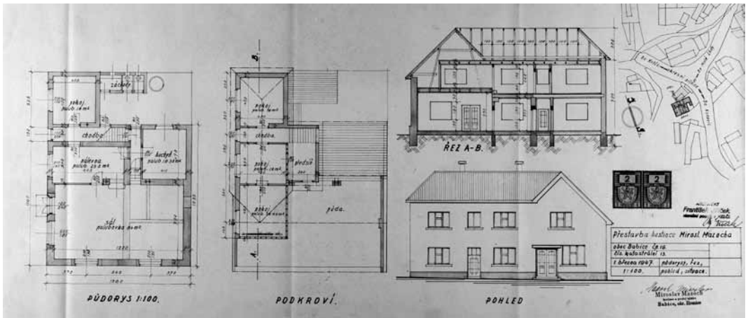
Stavební plán na přestavbu hostince v Babicích z roku 1947. SOkA Přerov, fond Okresní úřad Hranice, inv. č. 1445, kart. č. 793
