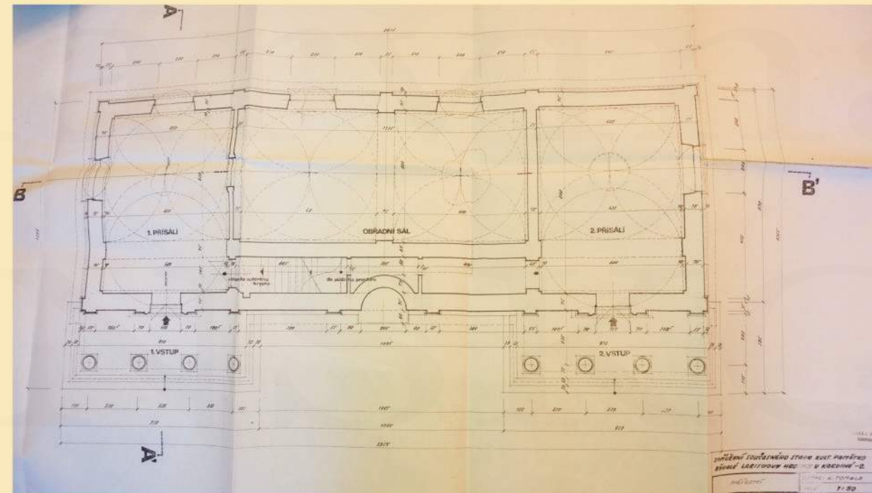
Ukázka dokumentace ze souboru dispozičních schémat zpracovaných K. Tomalou v roce 1980 pro TS Karviná (Magistrát města Karviná)
