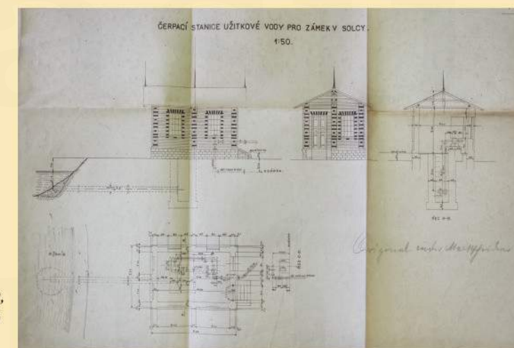
Plán z roku 1906 na stavbu čerpací stanice, která byla postavena v blízkosti zámeckého rybníku (Foto Petr Bindač, archiv OKD)
