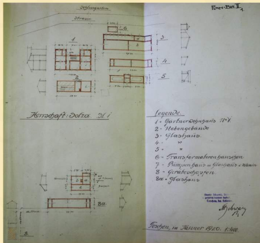
Popis objektů zámeckého zahradnictví: č. 1 – dům pro zaměstnance zahradnictví, č. 2 – přístavba, č. 3, 4, 5 – skleníky, č. 6 – trafostanice, č. 7 – rozvod vody pro potřeby skleníků, č. 8 – sklad nářadí, 8a – skleníky, rok 1920 (Foto Petr Bindač, archiv OKD)
