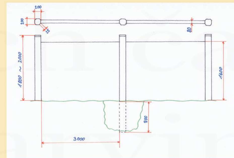
Rozměrový náčrtek betonového oplocení (autor nákresu: Petr Bindač)
