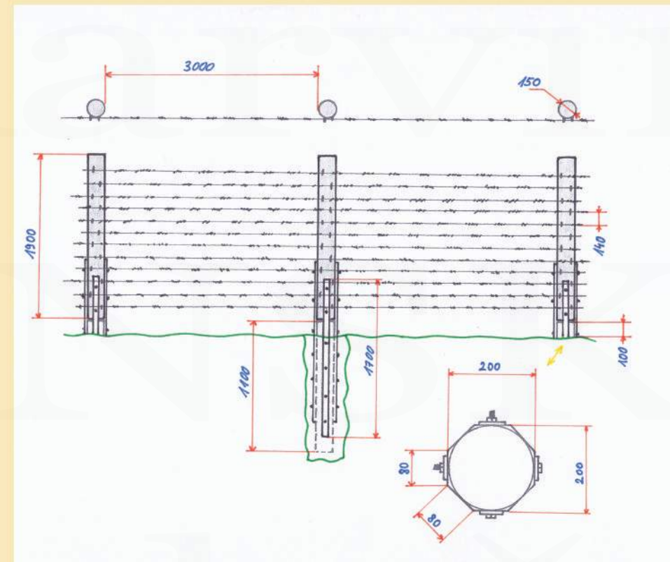
Rozměrový náčrtek oplocení ve spodní části parku (autor nákresu: Petr Bindač)
