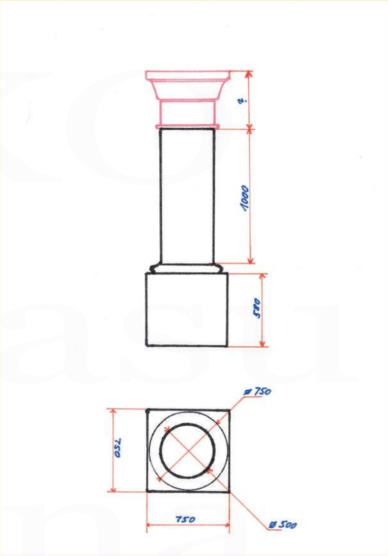
Rozměrový náčrtek sloupu z promenády (autor nákresu: Petr Bindač)
