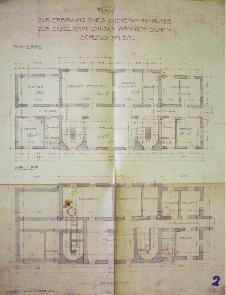
Plán na výstavbu domu pro služebnictvo z roku 1910 (Foto Petr Bindač, archiv OKD)
