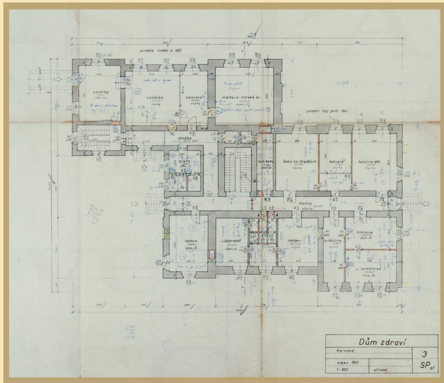
Plán adaptace přízemní části. Srpen 1947 (Foto Petr Bindač, archiv OKD)
