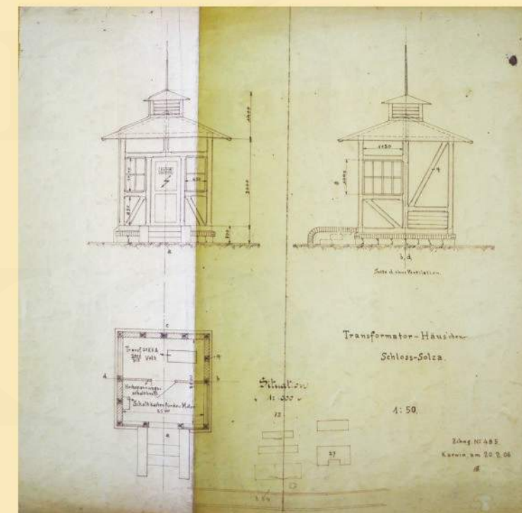
Plán z roku 1906 na výstavbu trafostanice, která poté stála v blízkosti zámeckého zahradnictví (Foto Petr Bindač, archiv OKD)
