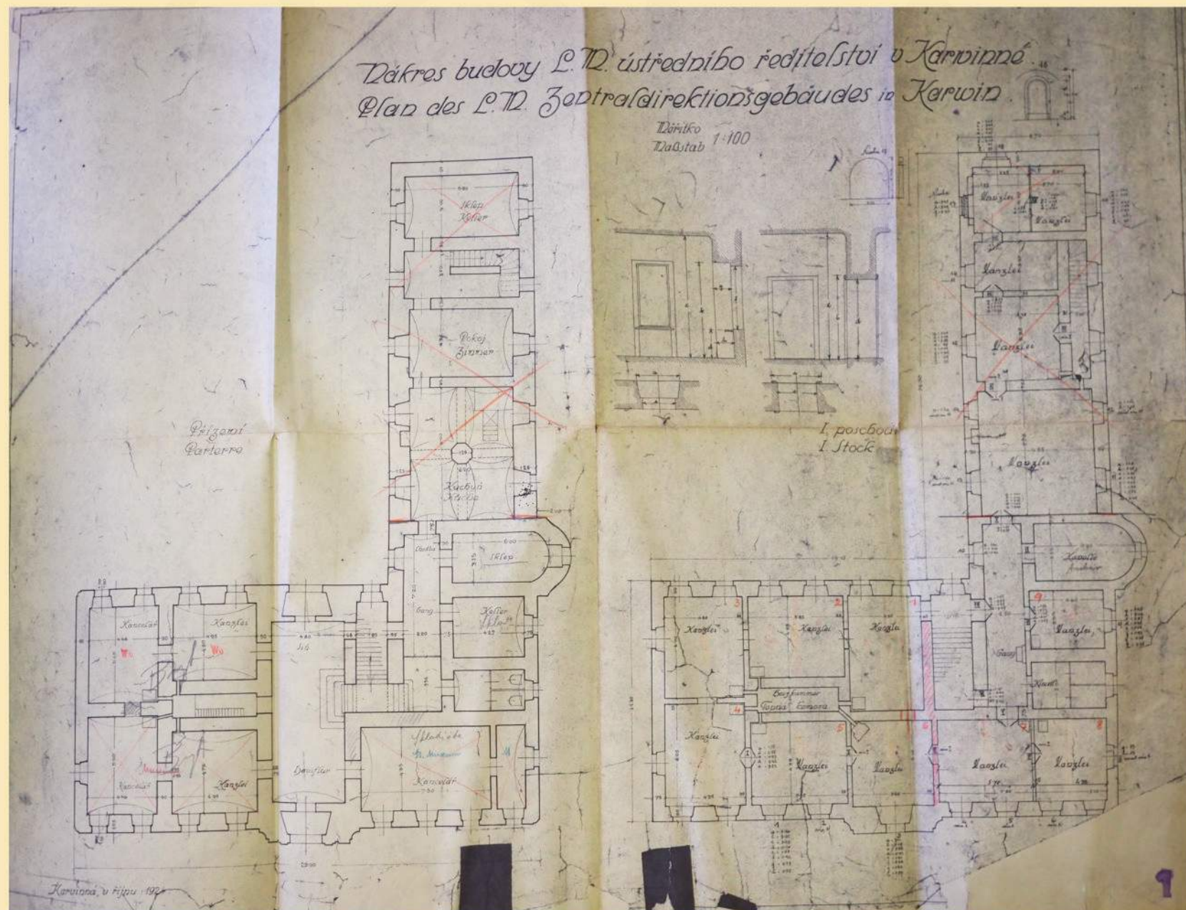
Nákres budovy z října 1924, ve kterém jsou dodatečně červeně zakresleny plánovaná demolice a úprava křídla (Archiv OKD, foto Petr Bindač)
