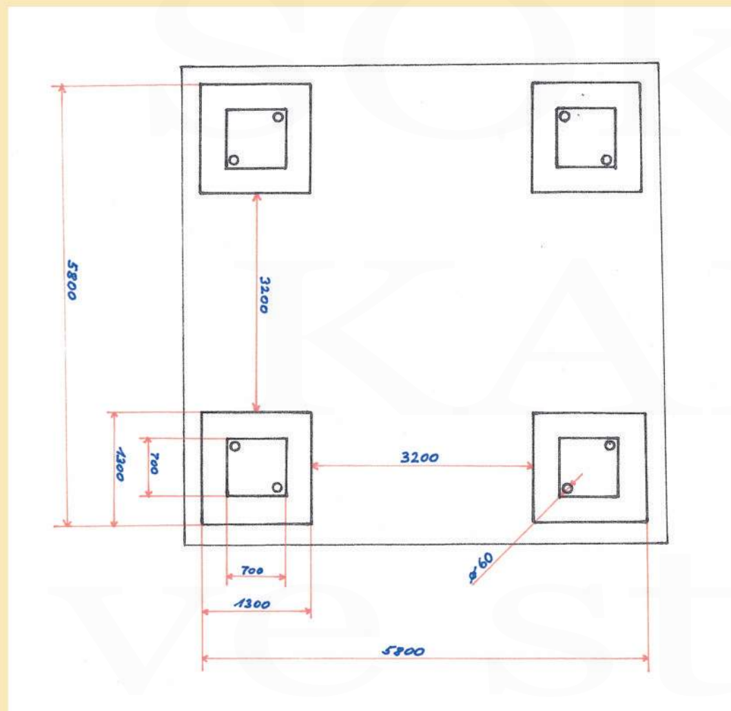
Rozměrový náčrtek dochovaných podstavců příhradové konstrukce hvězdy. Zaměření bylo provedeno na podzim 2021 (autor nákresu: Petr Bindač)
