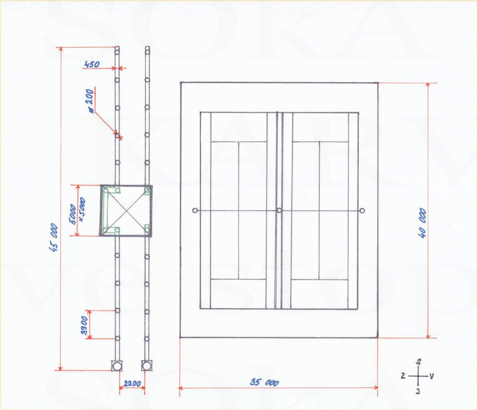
Rozměrový náčrtek promenády s tenisovými kurtů (autor nákresu: Petr Bindač)
