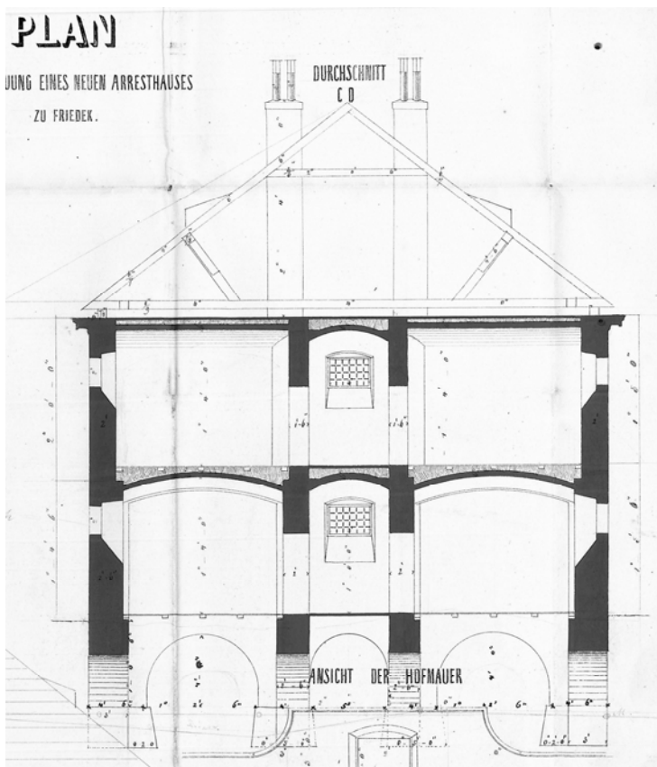
Svislý řez budovou věznice
