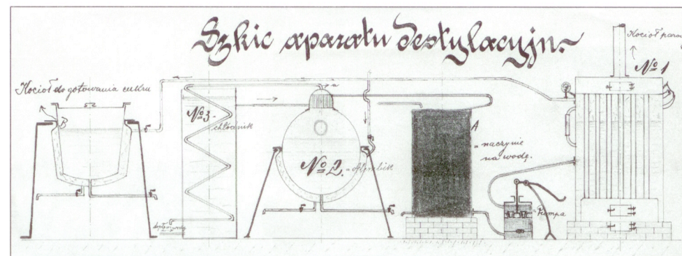
Náčrt destilačního přístroje.
