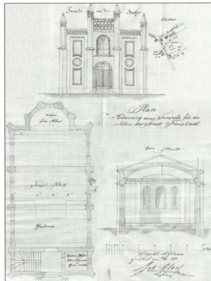
Stavební plán židovského templu z roku 1871.
