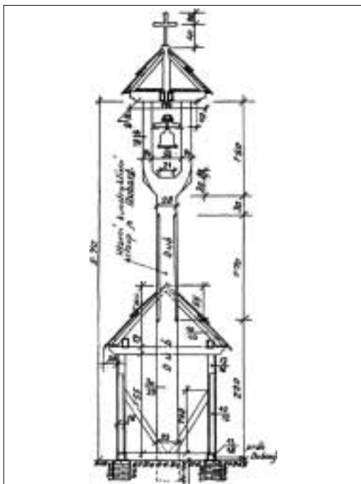
Obr. 9c. Plánek zvoničky v Zákřově. Archiv autora.
